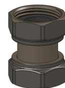
Rac diritto f-f con girello e guarnizione piana Female/female straight fitting with loose nut and flat seal
