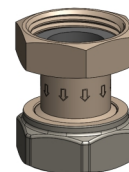
Rac diritto f-f con girello, guarnizione piana e valvola di non ritorno Female/female straight fitting with loose nut, flat seal and check valve
