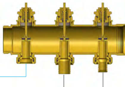
ART. 1859 Adattatore per trasformare attacco 1" G in battuta piana Adapter to have a plain on a 1" G connection
